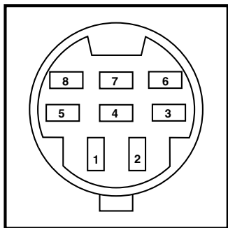
[32] Złącze szeregowe
